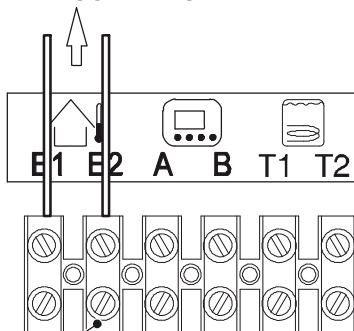
Morsettiera collegamento sonda esterna Figura 5.44
