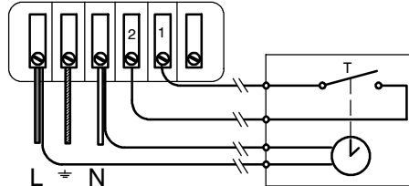
fig. 3.11 Termostato a due fili con orologio
