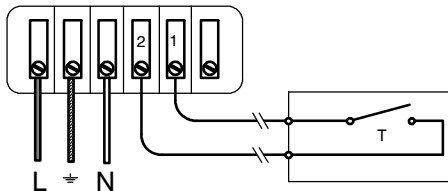
fig. 3.10 Termostato a due fili.
