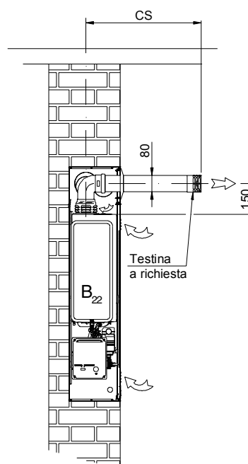
ASPIRAZIONE E SCARICO DIRETTAMENTE ALL'ESTERNO
