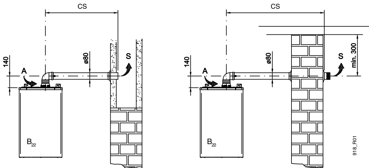
KIT FUMI PER ESTERNI
