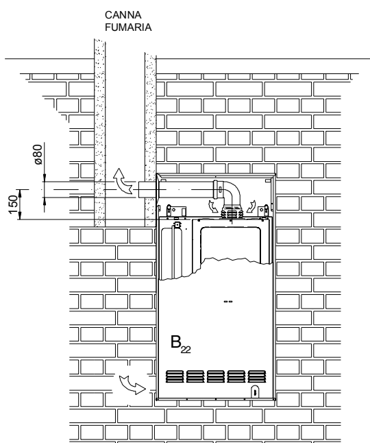
ASPIRAZIONE DIRETTAMENTE ALL'ESTERNO E SCARICO IN CANNA FUMARIA
