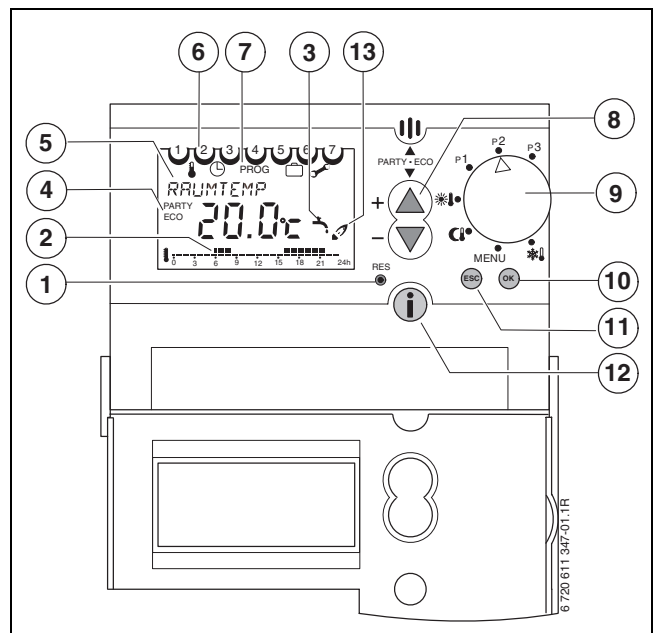
Fig. 8 Schema degli elementi di comando
