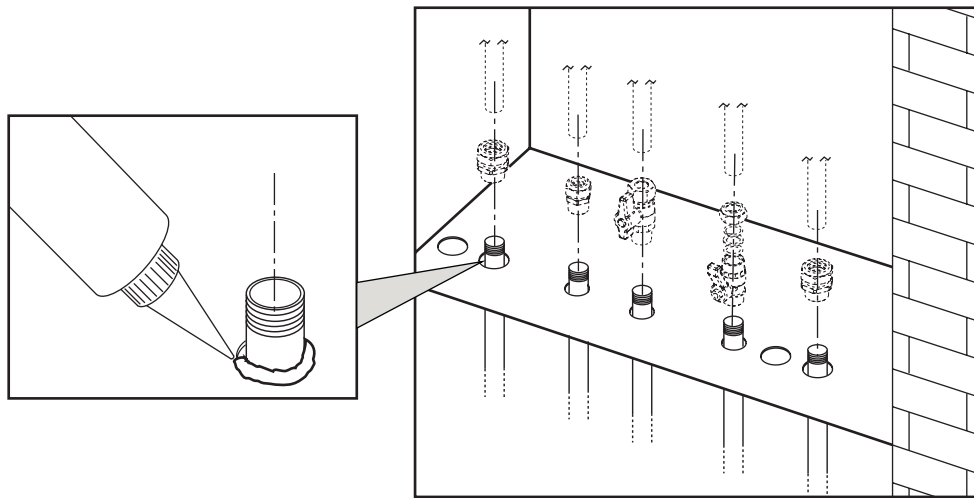
fig. 20 - Sigillatura involucro
