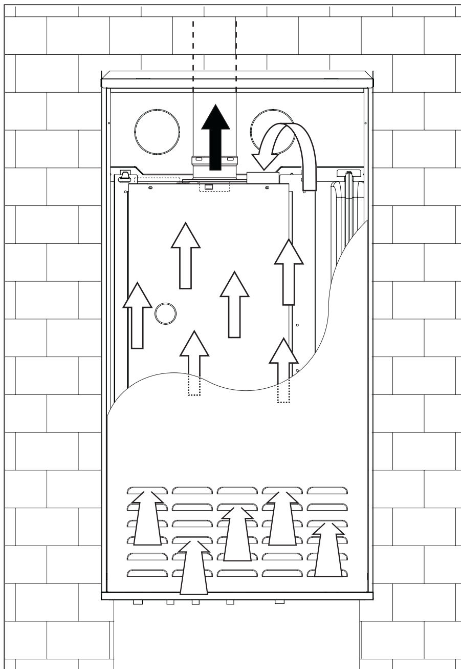
fig. 26 - Prelievo aria
