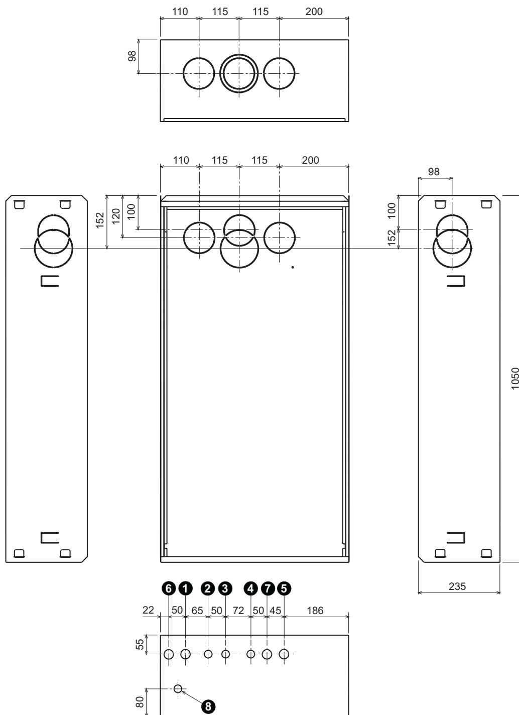
fig. 33 - Dimensioni e attacchi
