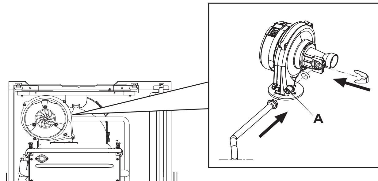
fig. 29 - Sostituzione ugello gas
