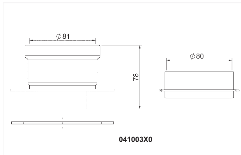
fig. 25 - Accessorio di partenza per condotti separati
