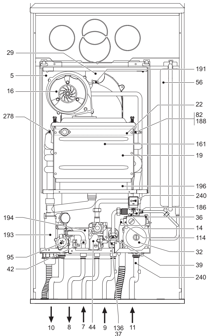
fig. 34 - Vista generale
