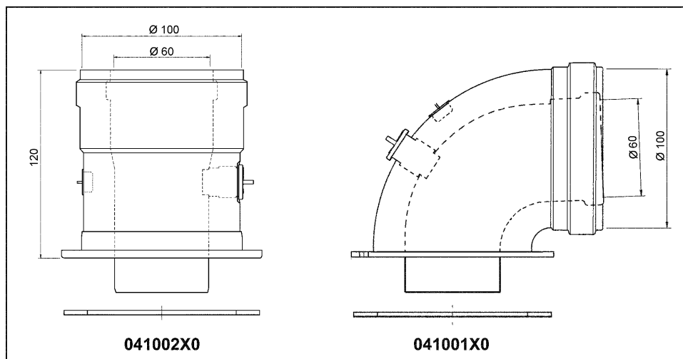
fig. 23 - Accessori di partenza per condotti coassiali
