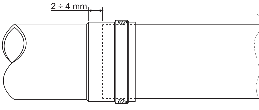
fig. 21 - Dilatazione
