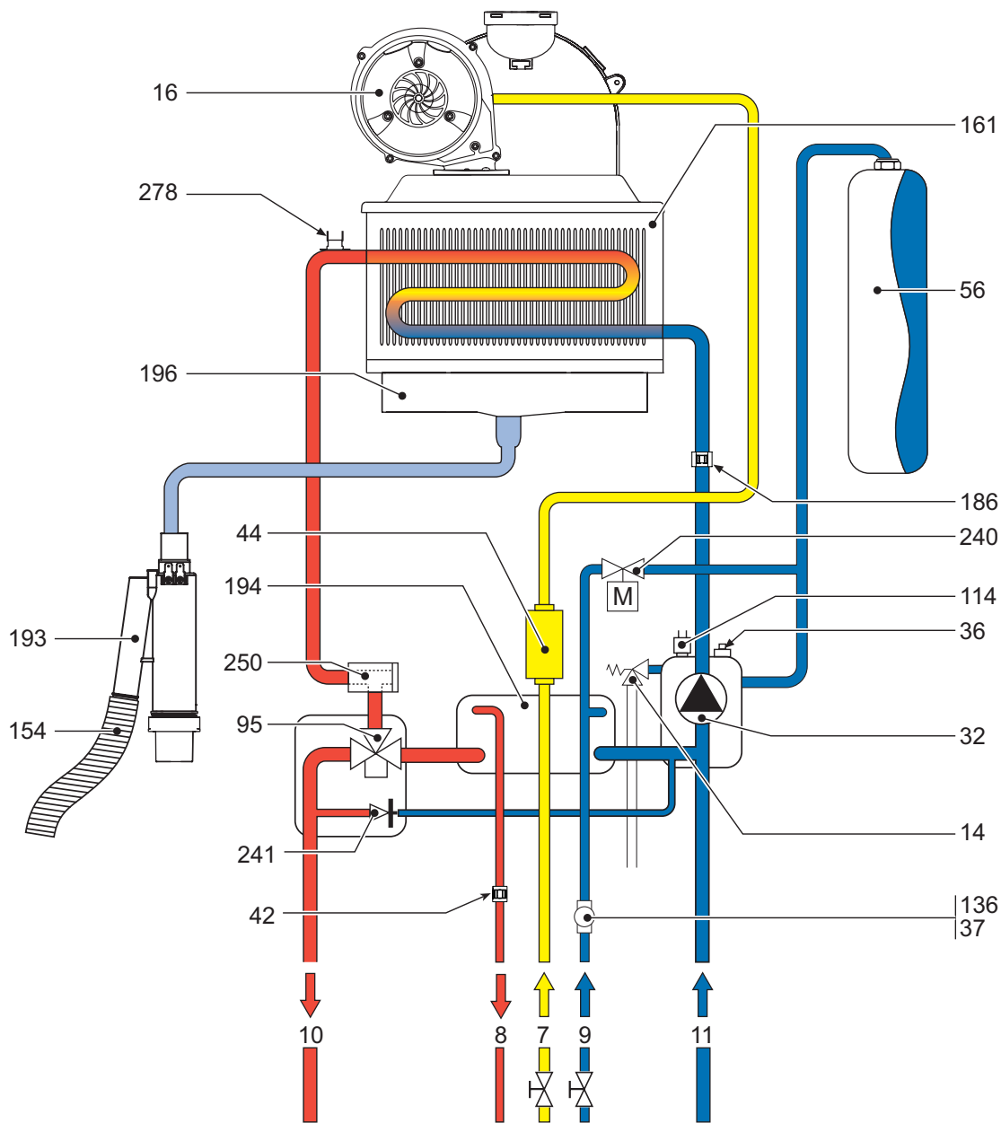
fig. 35 - Circuito idraulico
