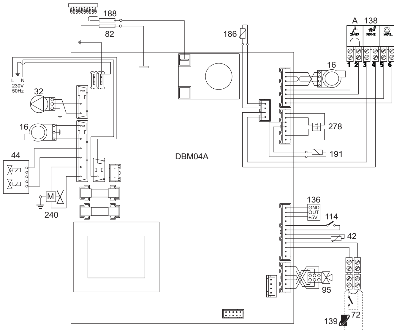
fig. 36 - Schema elettrico
