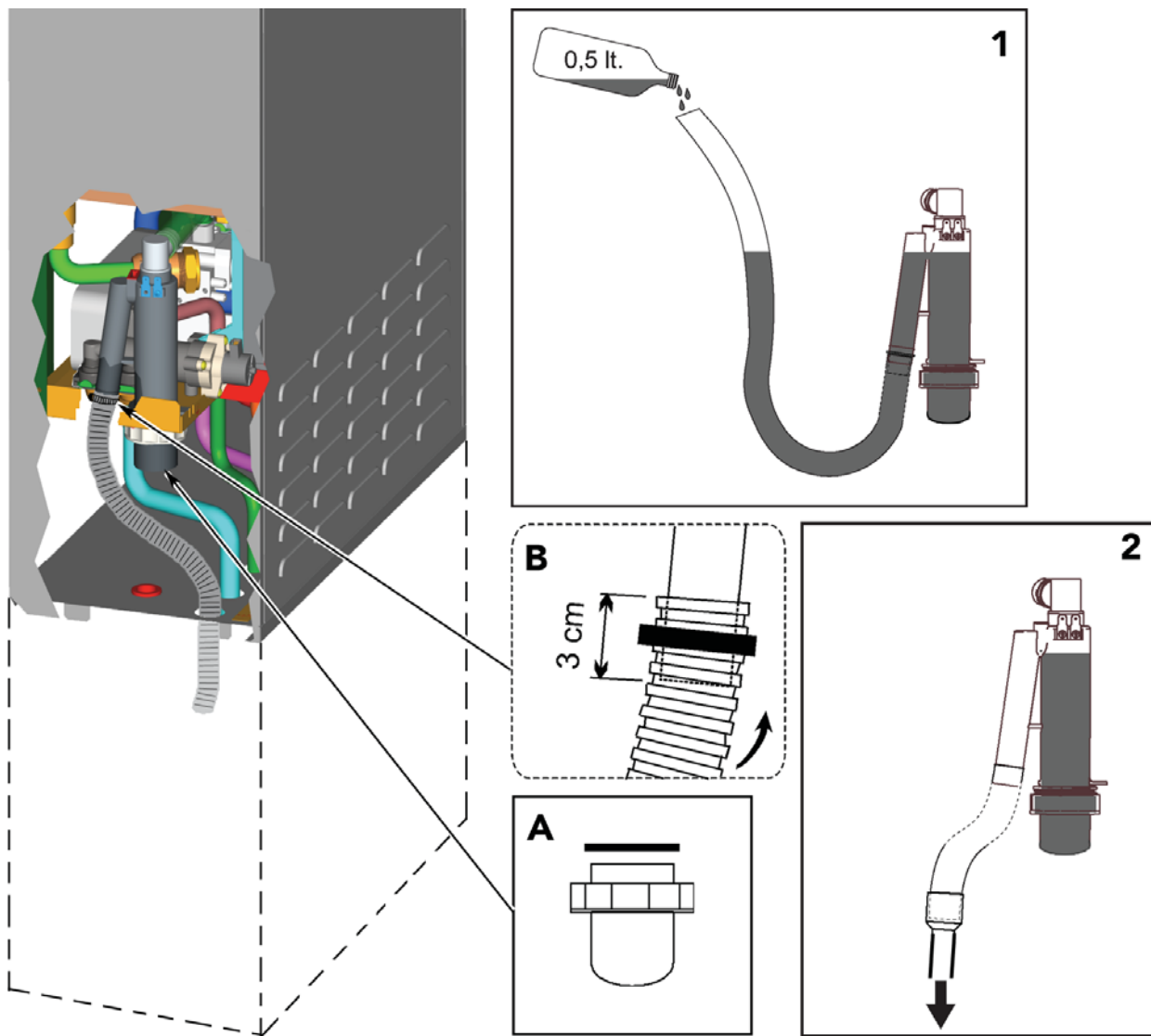
fig. 28 - Scarico condensa
