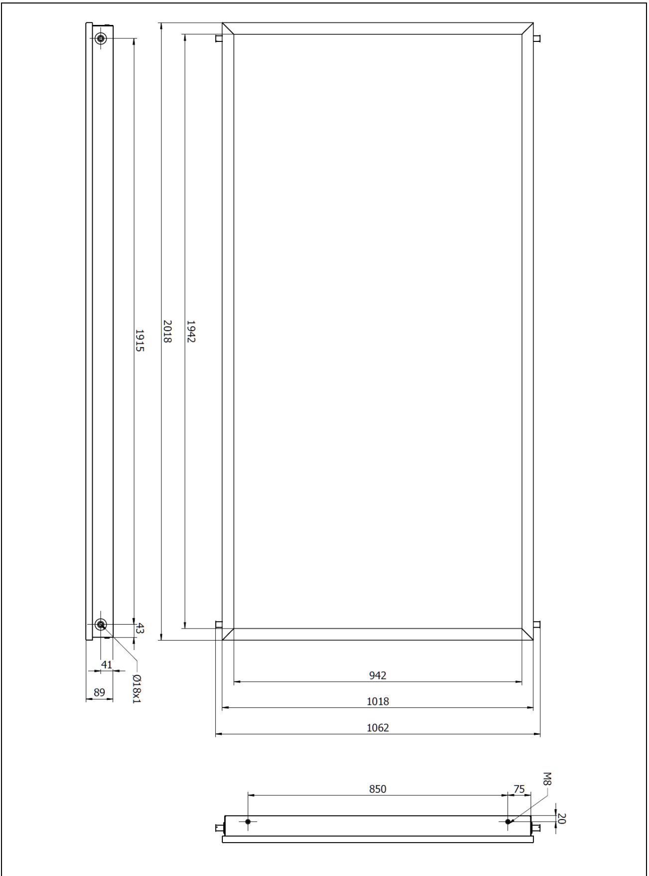
fig. 18 - Dimensions (mm)
