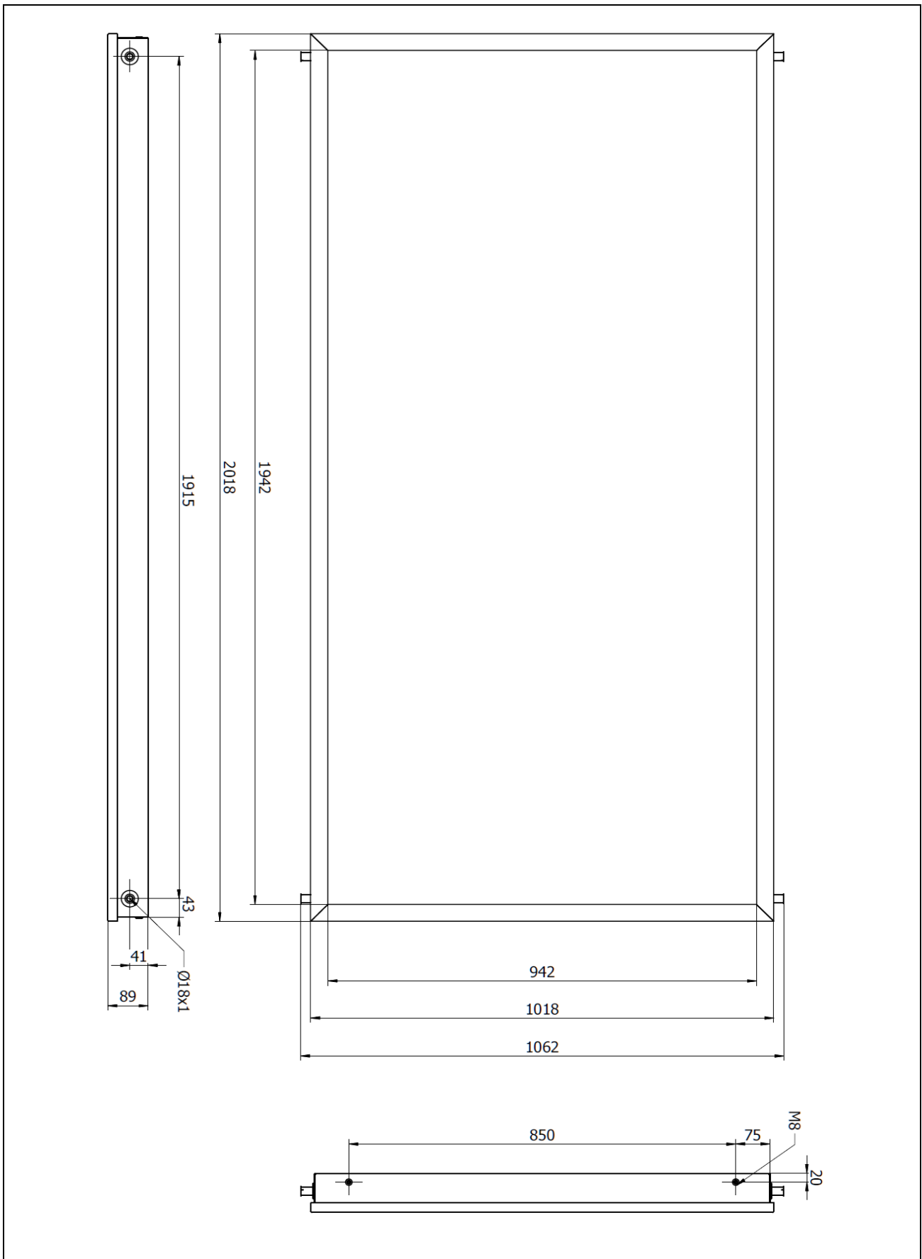
fig. 2 - Dimensioni (mm)
