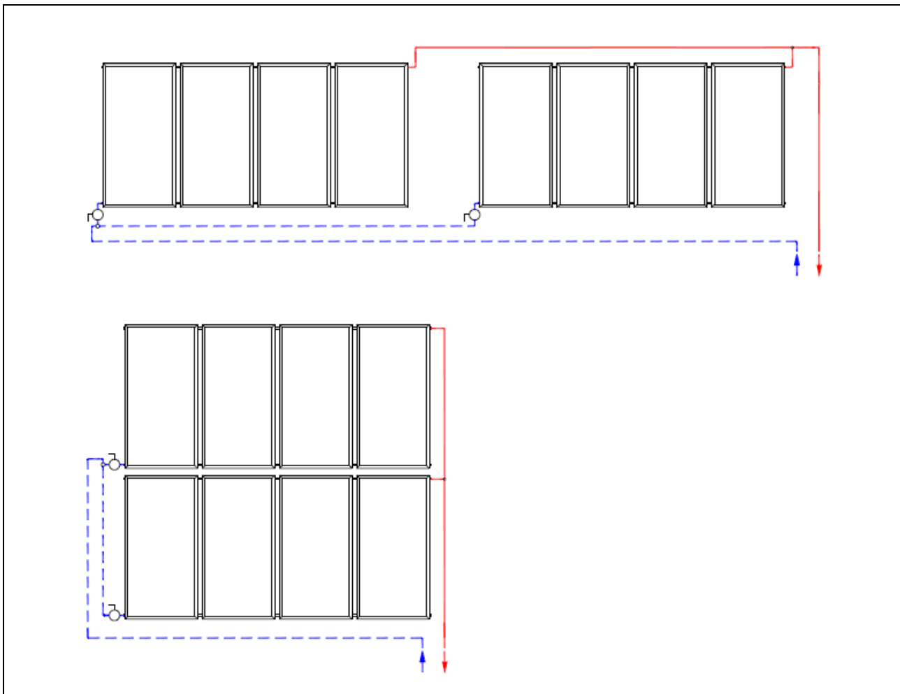
fig. 7 - Esempi di campi di collettori in serie-parallelo
