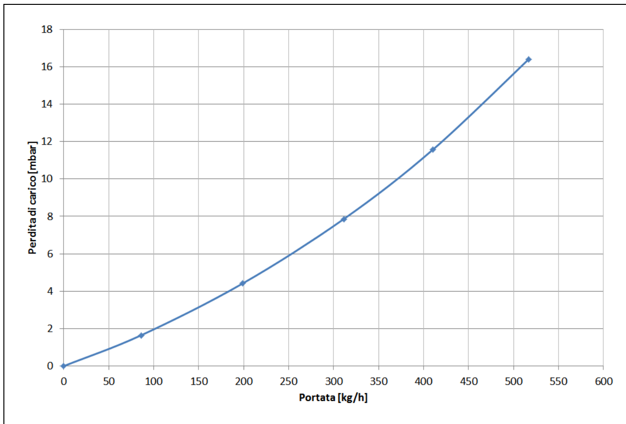
fig. 3 - Perdite di carico
