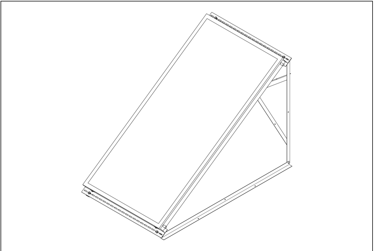
fig. 11 - Installazione su tetto piano con inclinazione di 35°
