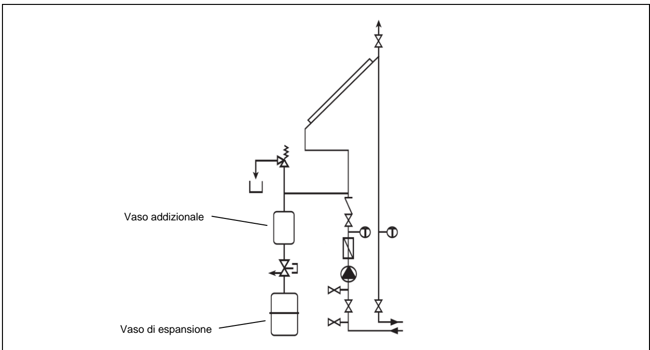
fig. 16 - Vaso di espansione
