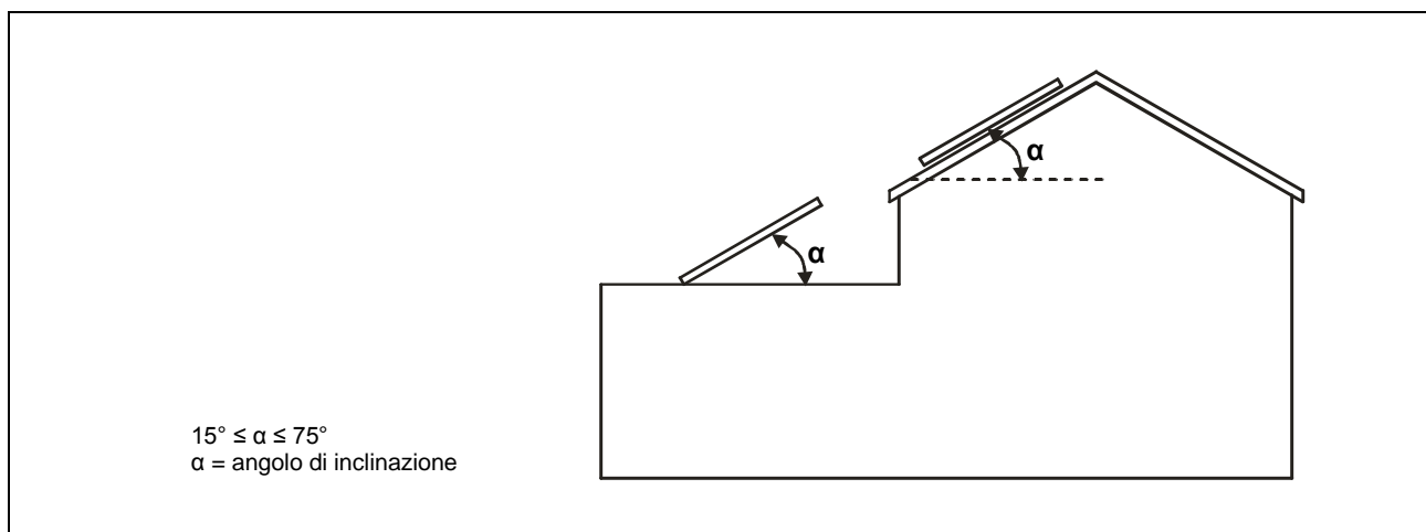
fig. 4 - Inclinazione dei collettori
