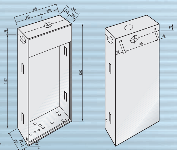
MISURE DI INGOMBRO TELAIO DI ALLOGGIAMENTO
