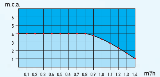
Diagramma portata prevalenza residua (con by-pass)
