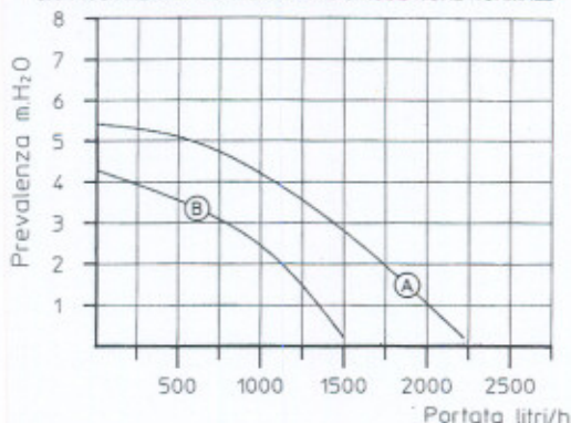
GRAFICO PREVALENZA DISPONIBILE CIRCOLATORE ALTA PREVALENZA
