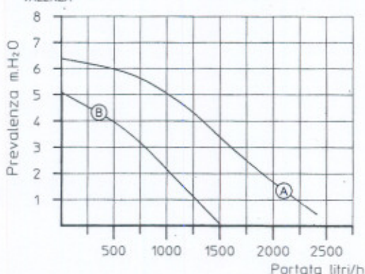
GRAFICO PREVALENZA DISPONIBILE CIRCOLATORE ALTA PREVALENZA
