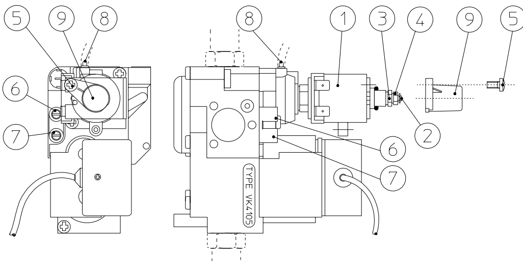
Valvola VK 4115 per Zeus Eco
