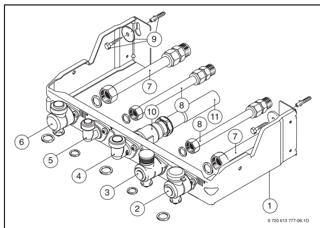
Fig. 10 Piastra d'installazione, accessorio nr. 893/18
