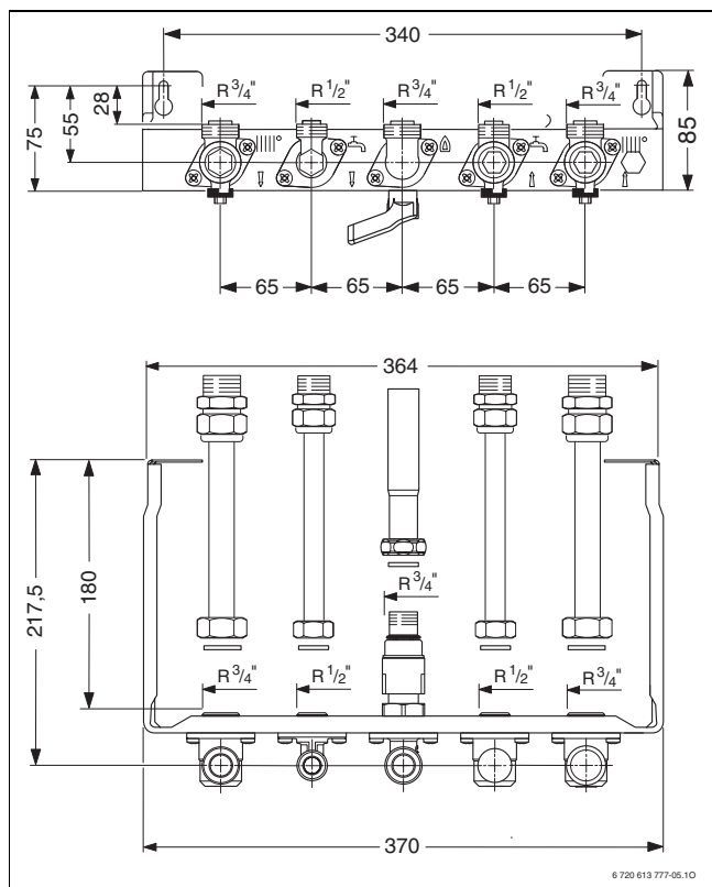
Fig. 9 Tubazioni a vista, realizzate in rame con brasatura piastra d'installazione, acc. nr. 893/18
