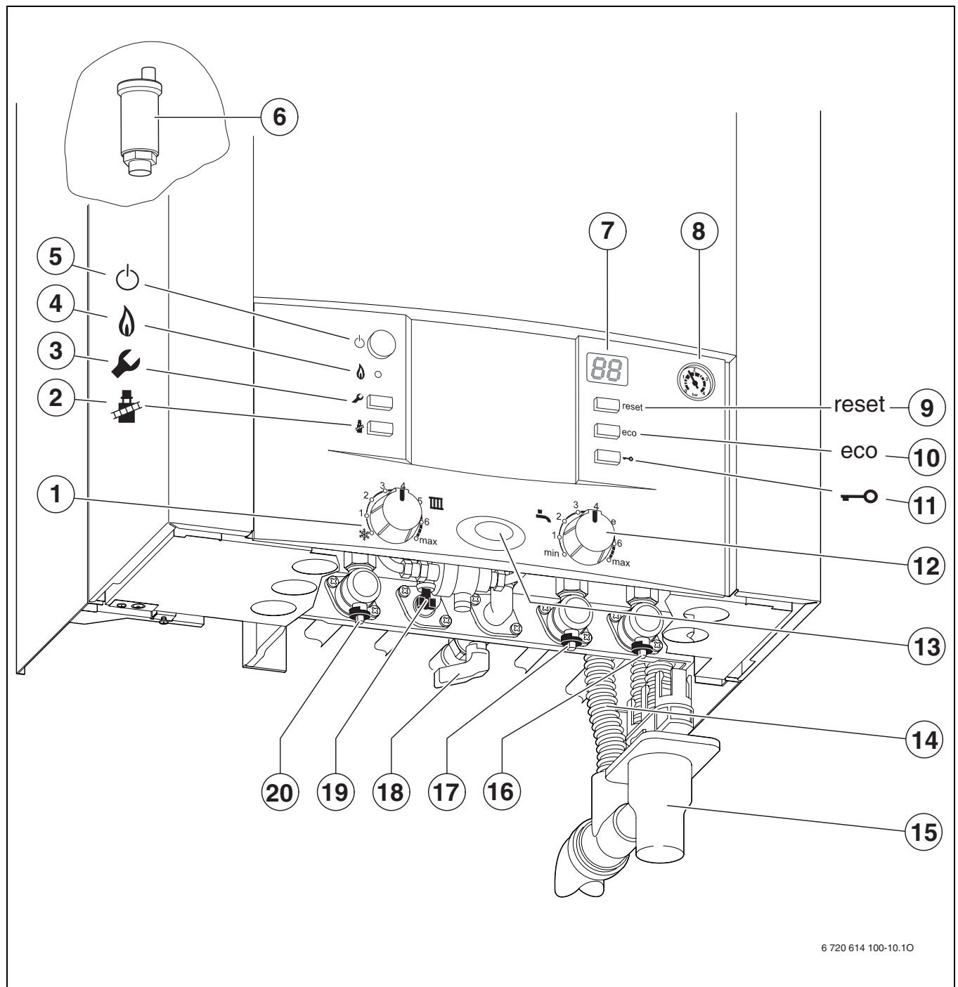
Fig. 26 Vista caldaia con accessorio nr. 893/18
