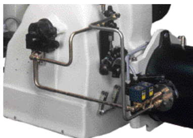
Gruppo valvole e camma a profilo variabile
