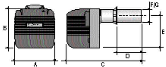
Apertura bruciatore ECO 22/2
