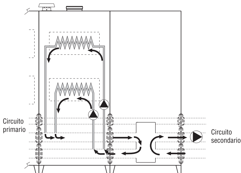
La pompa di circolazione impianto può anche essere alloggiata internamente all'armadio.
