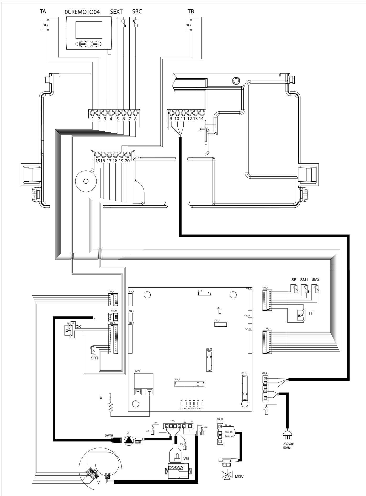
Fig. 25 Schema elettrico KRB
